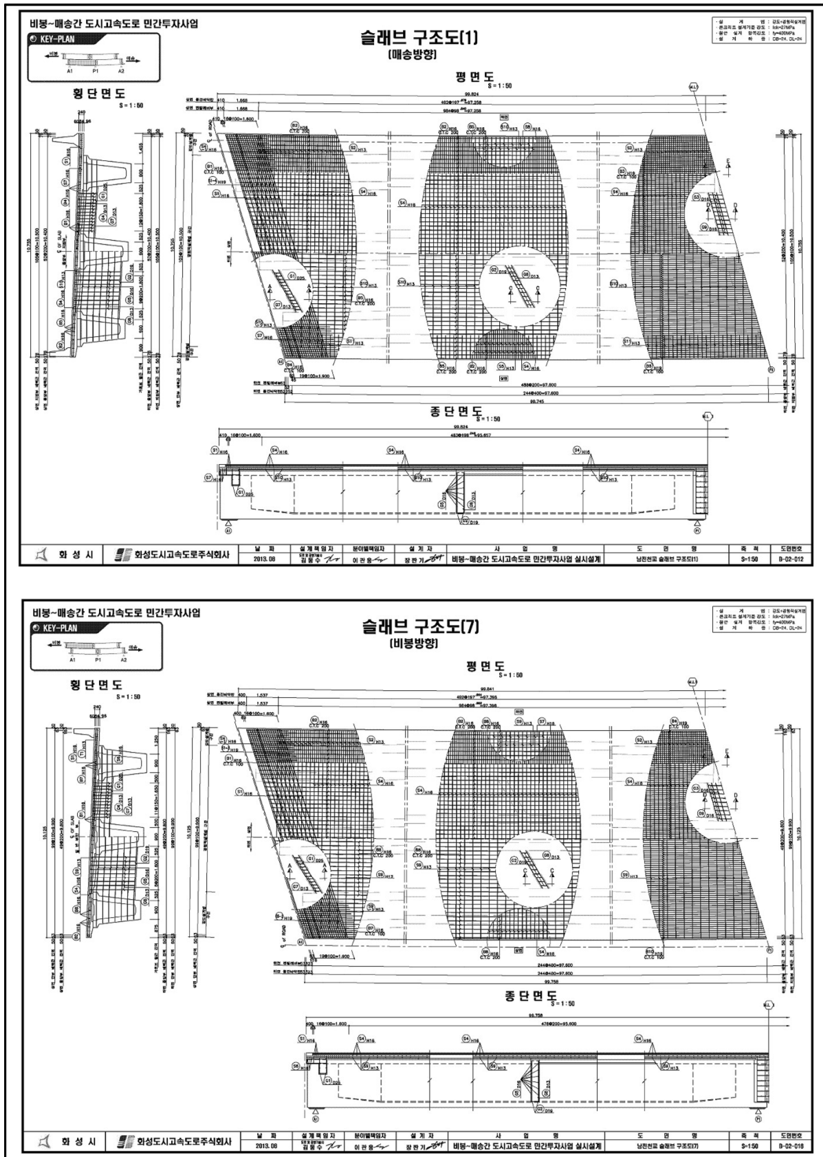
【그림 1.1.6】 슬래브 구조도
