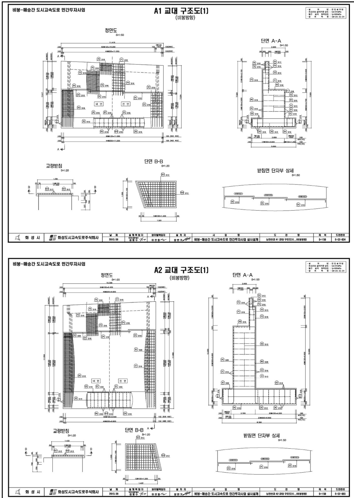
【그림 1.1.13】 교대 구조도(비봉방향)
