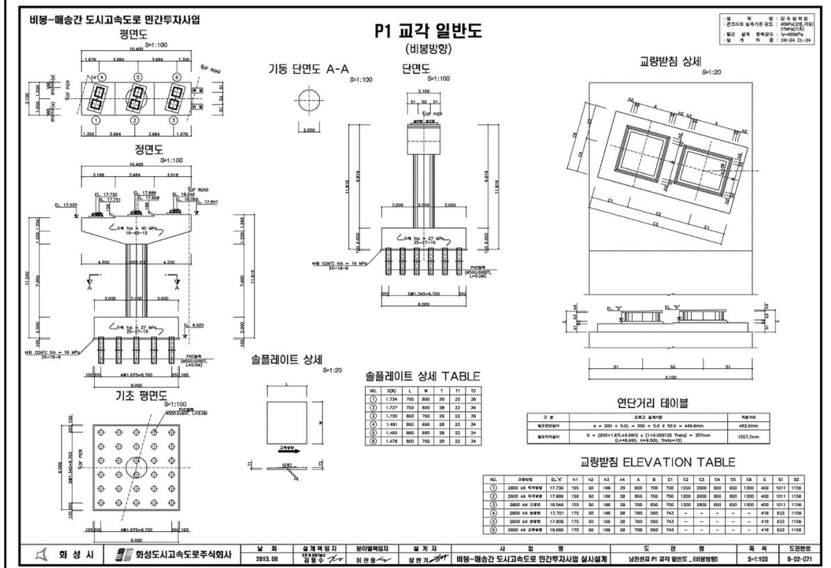
【그림 1.1.14】 교각 일반도
