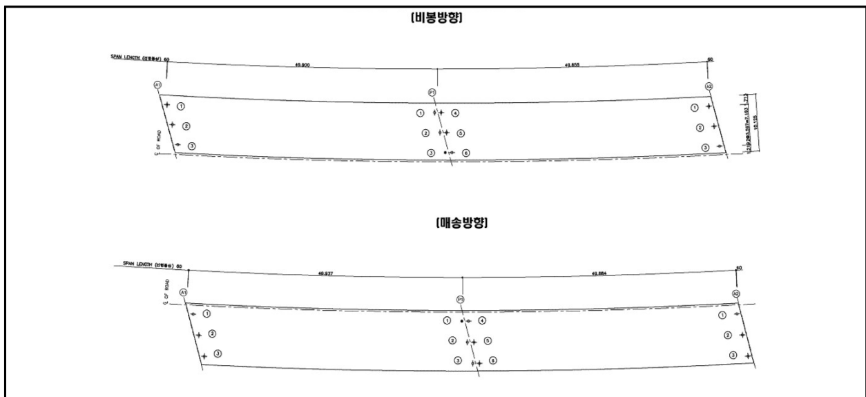
【그림 1.3.3】 교량받침 배치도
