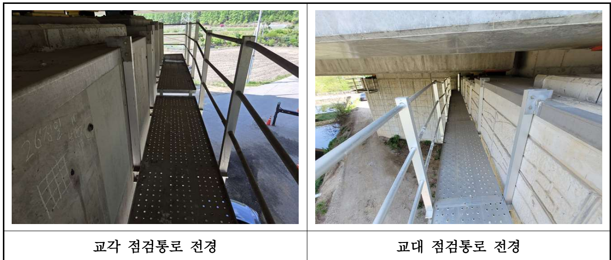
【사진 1.3.29】 교량 점검시설 전경
